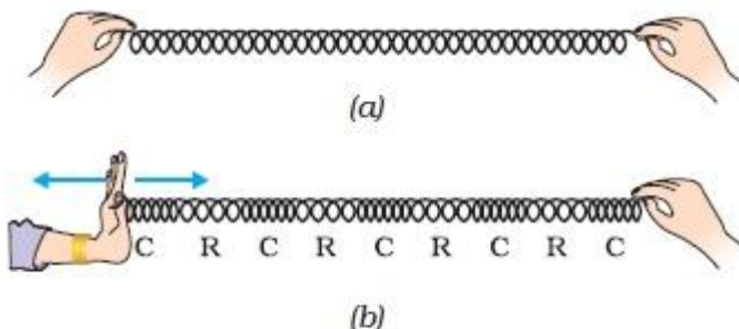
Fig. 12.7: Longitudinal wave in a slinky.
