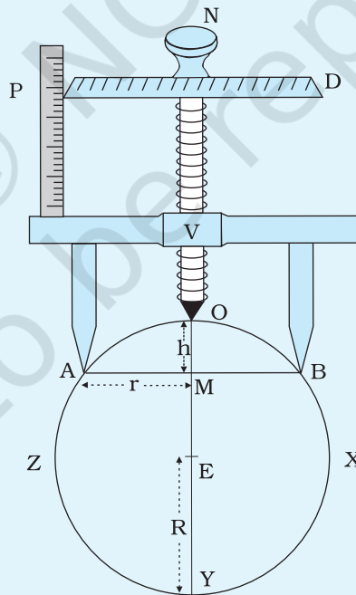
चित्र E 3.2 किसी गोलीय पृष्ठ के वक्रता अर्धव्यास का मापन
