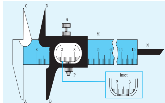
चित्र E 1.1 वर्नियर कैलिपर्स
