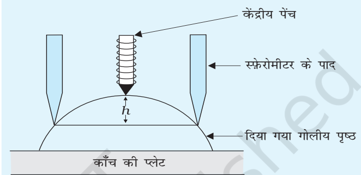
चित्र E 3.4 सैजिता h का मापन
