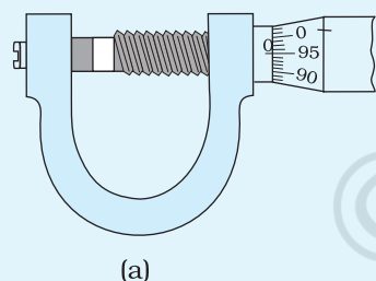
चित्र E 2.4 (a) धनात्मक शून्यांक त्रुटि की कोई स्थिति
