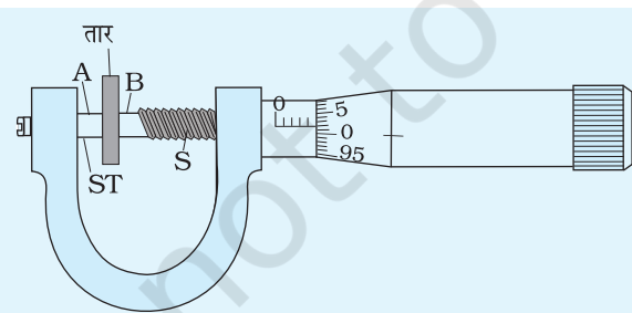
चित्र E 2.5 स्कूगेज से मोटाई मापना
