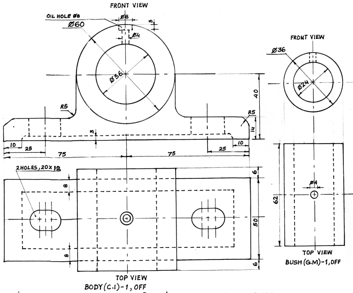
चित्र 1/FIG-1. BUSHED BEARING
